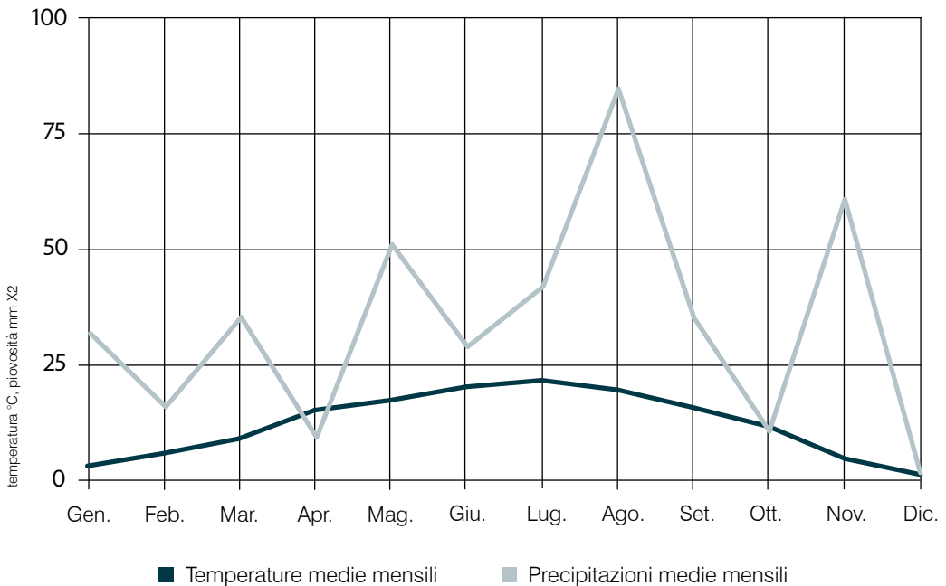
GRAFICO 19 - STAZIONE DI SAN MICHELE ALL'ADIGE: DIAGRAMMA DI GAUSSEN (2007)
