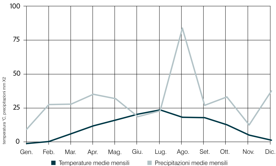
GRAFICO 18 - STAZIONE DI SAN MICHELE ALL'ADIGE: DIAGRAMMA DI GAUSSEN (2006)
