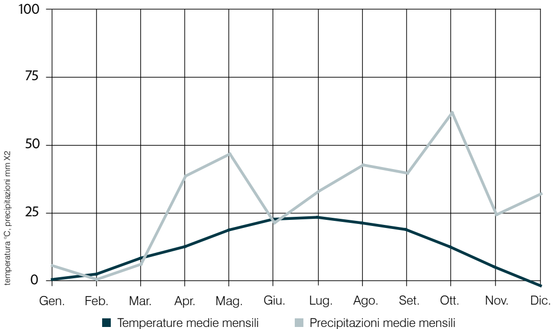
GRAFICO 17 - STAZIONE DI SAN MICHELE ALL'ADIGE: DIAGRAMMA DI GAUSSEN (2005)
