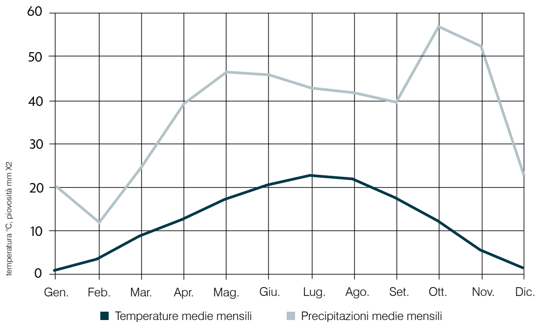
GRAFICO 20 - STAZIONE DI SAN MICHELE ALL'ADIGE: CLIMOGRAMMA DI GAUSSEN (1983 - 2007)
