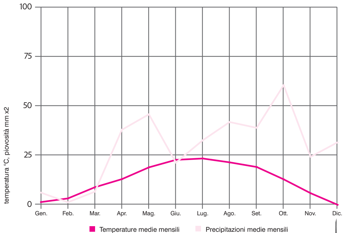
GRAFICO 19 - STAZIONE DI SAN MICHELE ALL'ADIGE: DIAGRAMMA DI GAUSSEN (2005)
