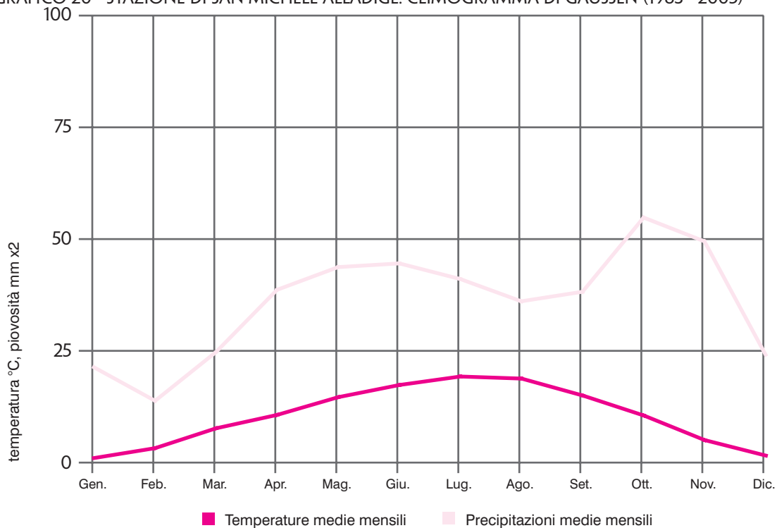
GRAFICO 20 - STAZIONE DI SAN MICHELE ALL'ADIGE: CLIMOGRAMMA DI GAUSSEN (1983 - 2005)
