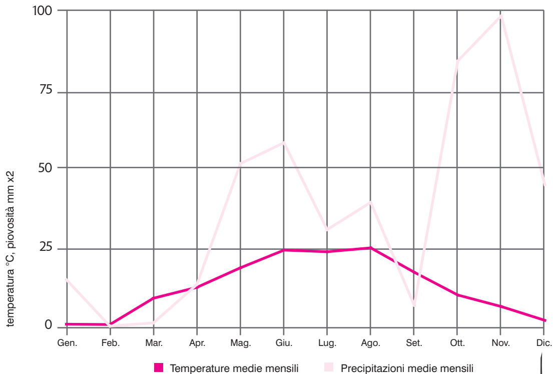
GRAFICO 17 - STAZIONE DI SAN MICHELE ALL'ADIGE: DIAGRAMMA DI GAUSSEN (2003)
