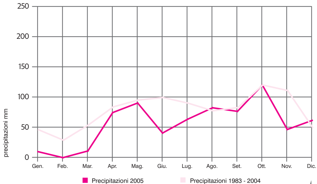
GRAFICO 22 - STAZIONE DI SAN MICHELE ALL'ADIGE: PRECIPITAZIONI 2005 A CONFRONTO CON LA MEDIA DELLE PRECIPITAZIONI (1983-2004)
