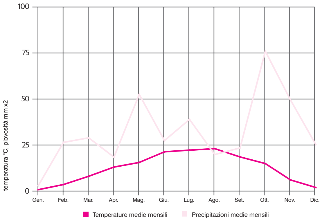
GRAFICO 18 - STAZIONE DI SAN MICHELE ALLADIGE: DIAGRAMMA DI GAUSSEN (2004)
