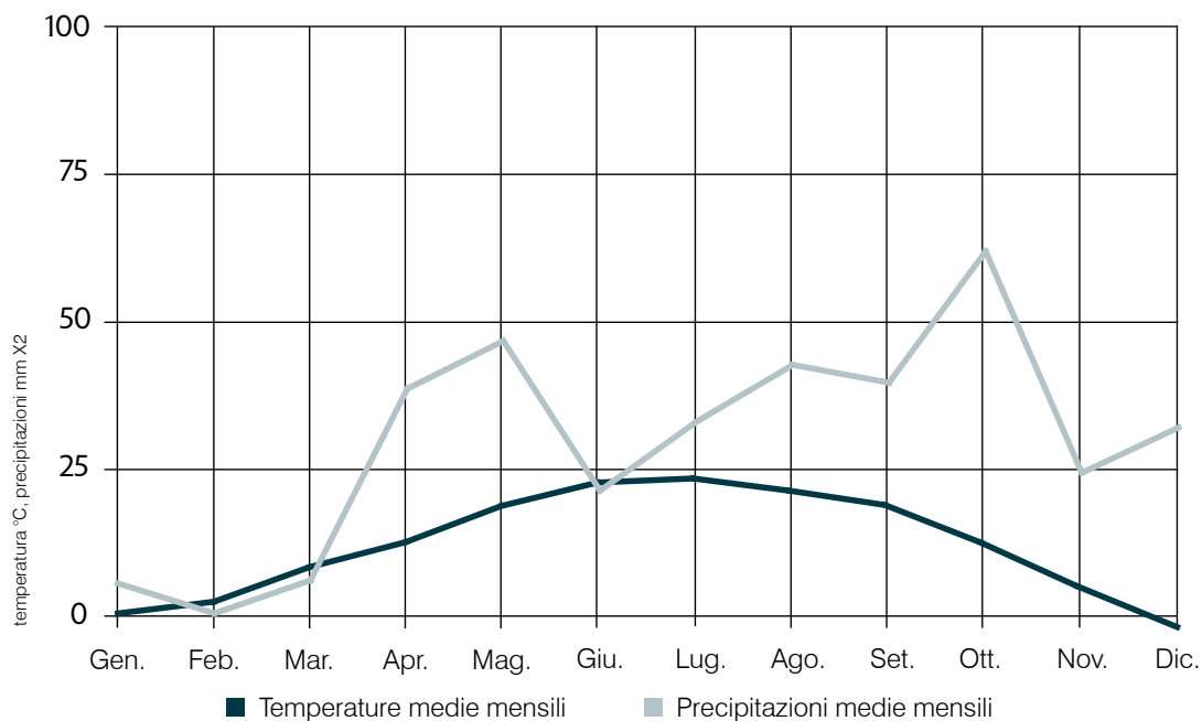
GRAFICO 17 - STAZIONE DI SAN MICHELE ALL'ADIGE: DIAGRAMMA DI GAUSSEN (2005)
